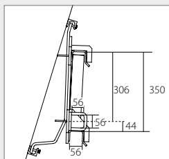
5. Schäffer-Hoflader mechanische Verriegelung Obere Einhängehöhe: 966 mm
