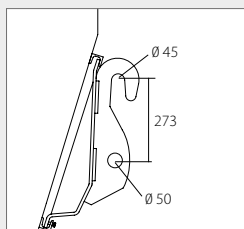
6. Kramer-Allrad Obere Einhängehöhe: 959 mm
