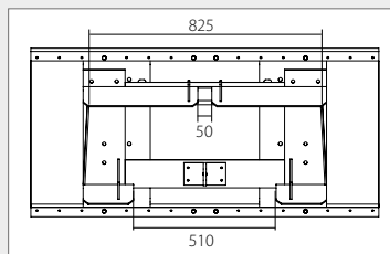
5. Schäffer-Hoflader mechanische Verriegelung Obere Einhängehöhe: 966 mm
