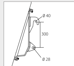
4. Euronorm Obere Einhängehöhe: 890 mm
