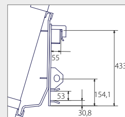
7. Thaler Obere Einhängehöhe: 966 mm
