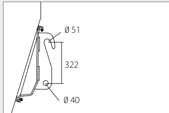
3. Weidemann hydraulische Verriegelung Obere Einhängehöhe: 915 mm
