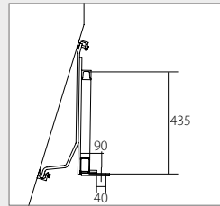
2. Weidemann mechanische Verriegelung Obere Einhängehöhe: 927 mm
